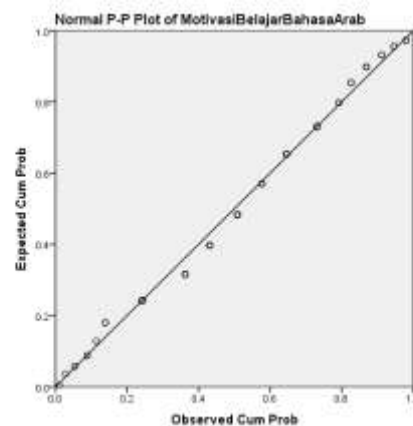
Grafik 4. 1 Grafik Normal P-P Plot
