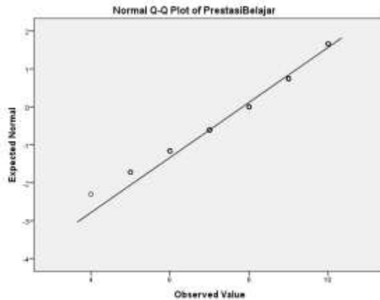
Gambar 4.3 Uji Normalitas Data Variabel dependen dengan QQ Plot
